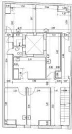
PLANTA PRIMERA
