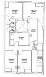
PLANTA PRIMERA SUPERF. DEL TOTAL 118,42 M 2 SUPERF. CONSTRUCHA 88,36 M 2
