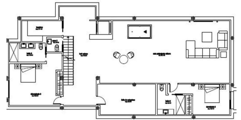
planta sótano
