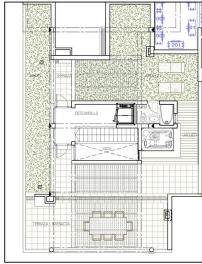
PLANTA TERRAZA - JARDIN
